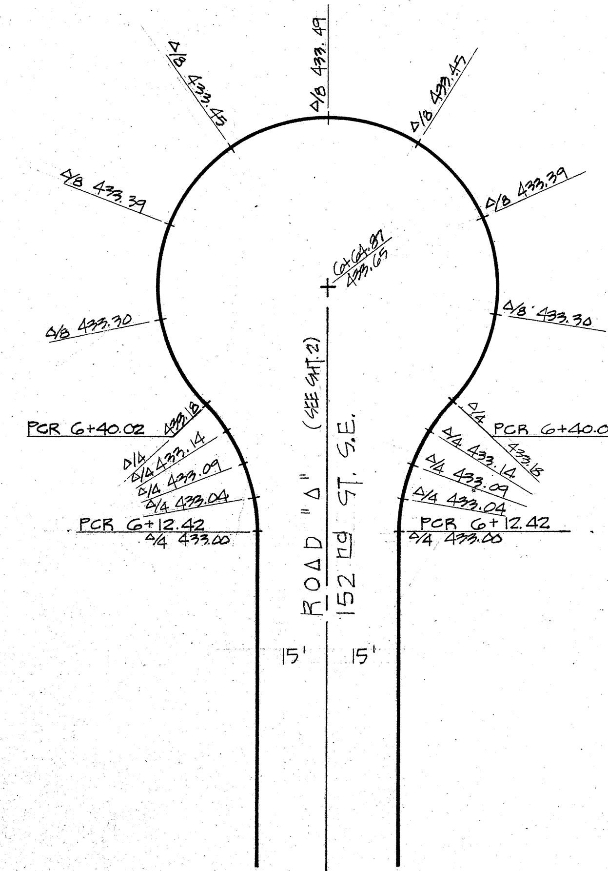
GUTTER GRADES @ 152 RD ST. S.E. CUL. DE SAC SCALE: 1" = 20'
