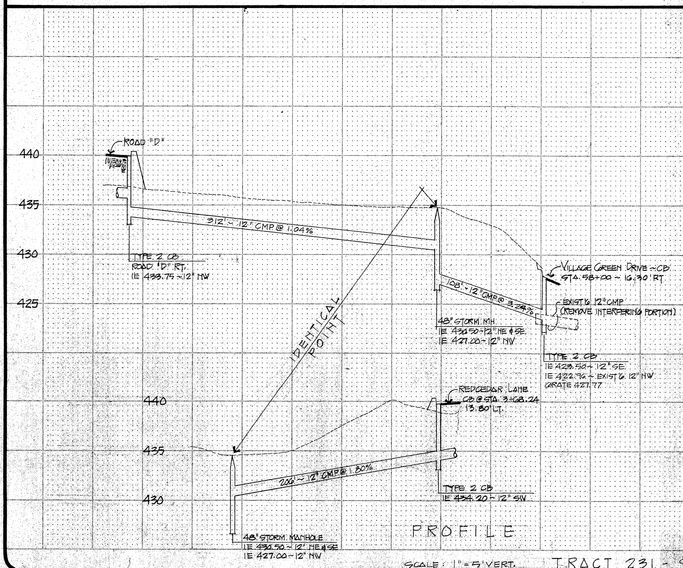
SCALE: 1" = 5' VERT.
